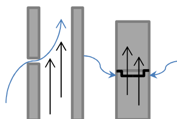
Figura 23 - Vedação incorreta
