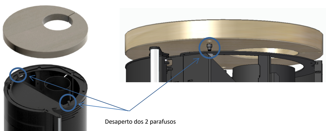
Figura 13 - Colocação do tampo em pedra no equipamento com saída de fumos na vertical
