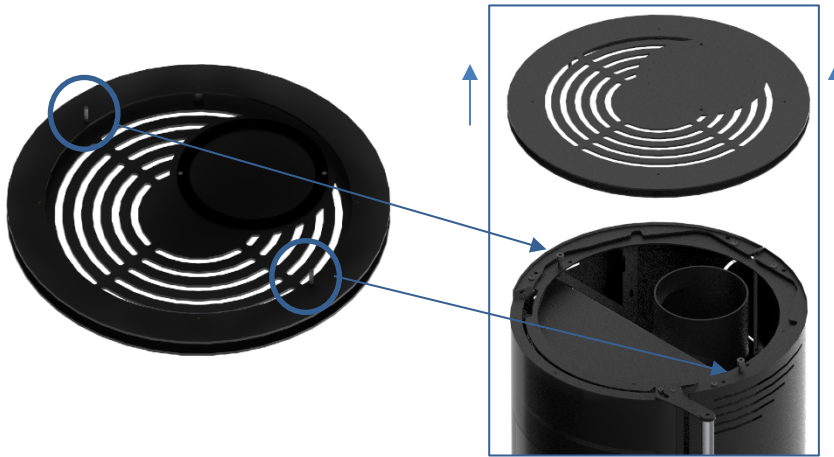
Figura 15 - Desmontagem do tampo no equipamento
