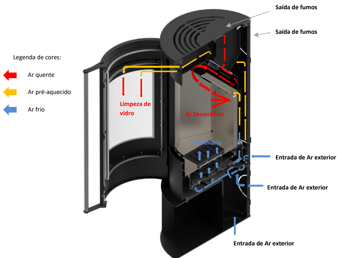
Figura 29 - Circuito de convecção representada na salamandra
