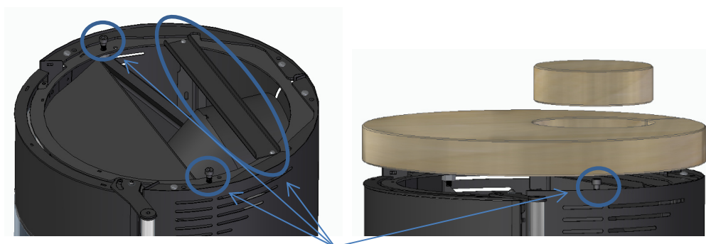
Figura 14 - Colocação do tampo em pedra no equipamento com saída de fumos na horizontal
