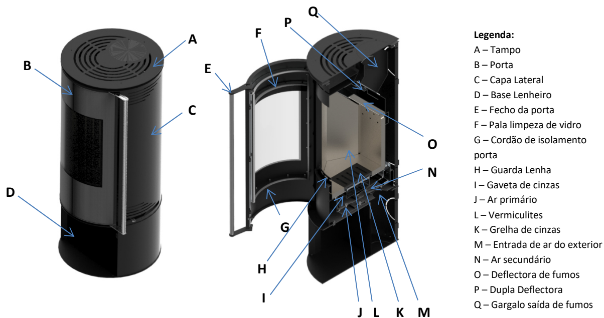
Figura 3 - Componentes da salamandra Amber
