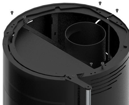
Figura 16 - Desmontagem das capas laterais no equipamento
