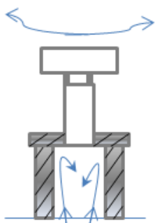
Figura 24 - União incorreta
